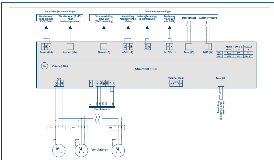
Aansluitschema TSC5-PCB met TSC5 (standaard voor W en LW)
