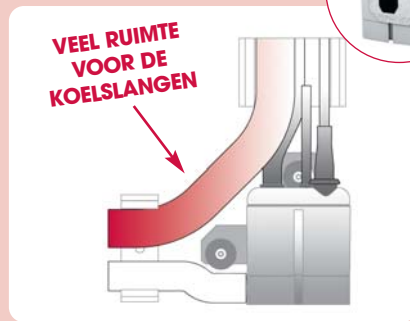
Voor de doorvoer van koelsslangen met een maximale diameter van 5/8" - 3/8"
